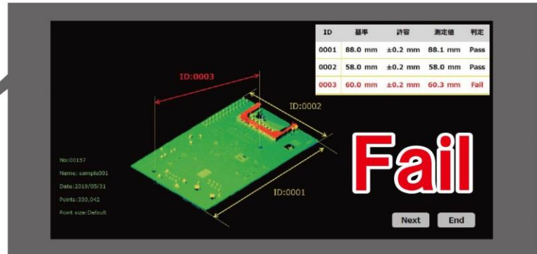
IDごとに基準値と3D計測値を自動で比較して合否判定
